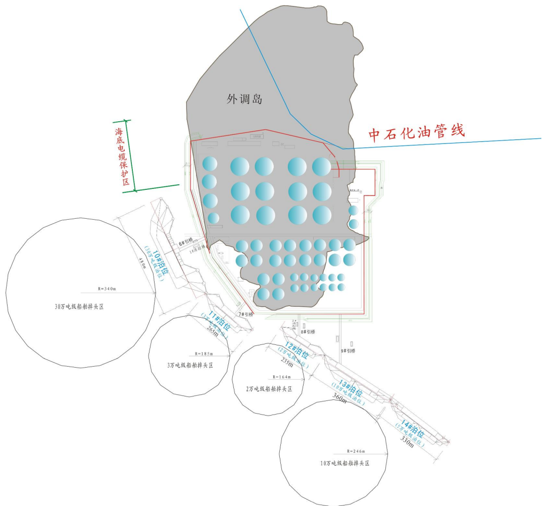
图 2-1 拟建码头平面布置图
